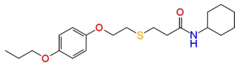
DUD-E 6
