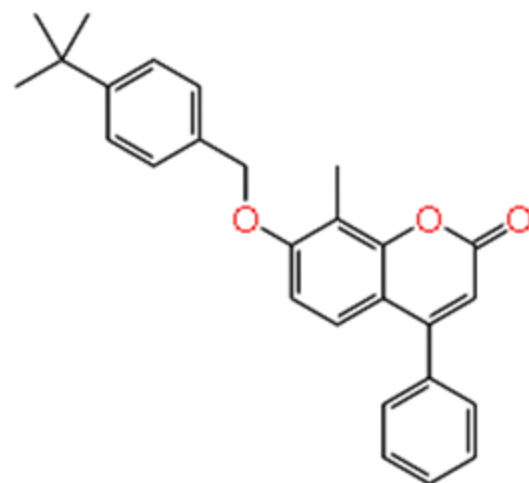
DUD-E 3
