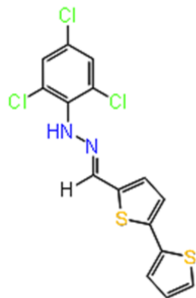
DUD-E 1
