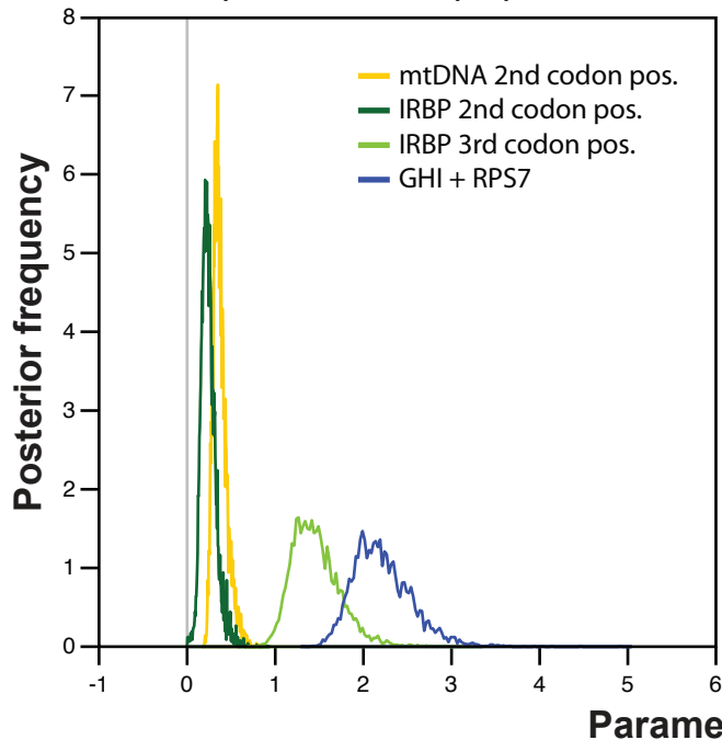
DNA partition \Gamma shape parameter
