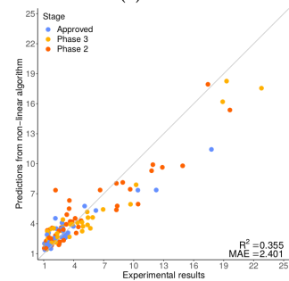
(f) BVP
