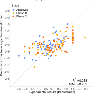
(d) ACSINS
