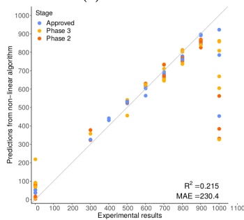
(g) SGAC-SINS
