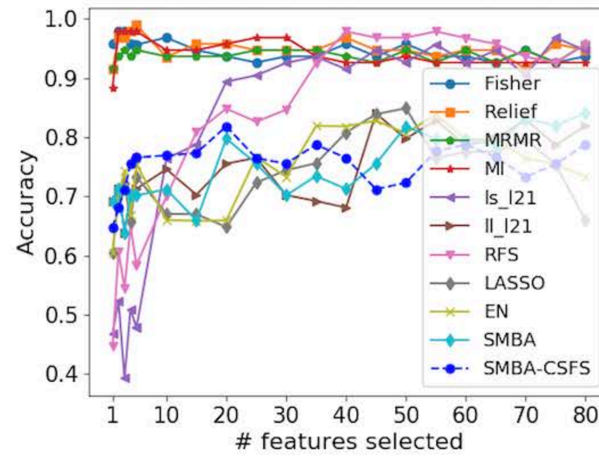
(b) LEUKEMIA (2)
