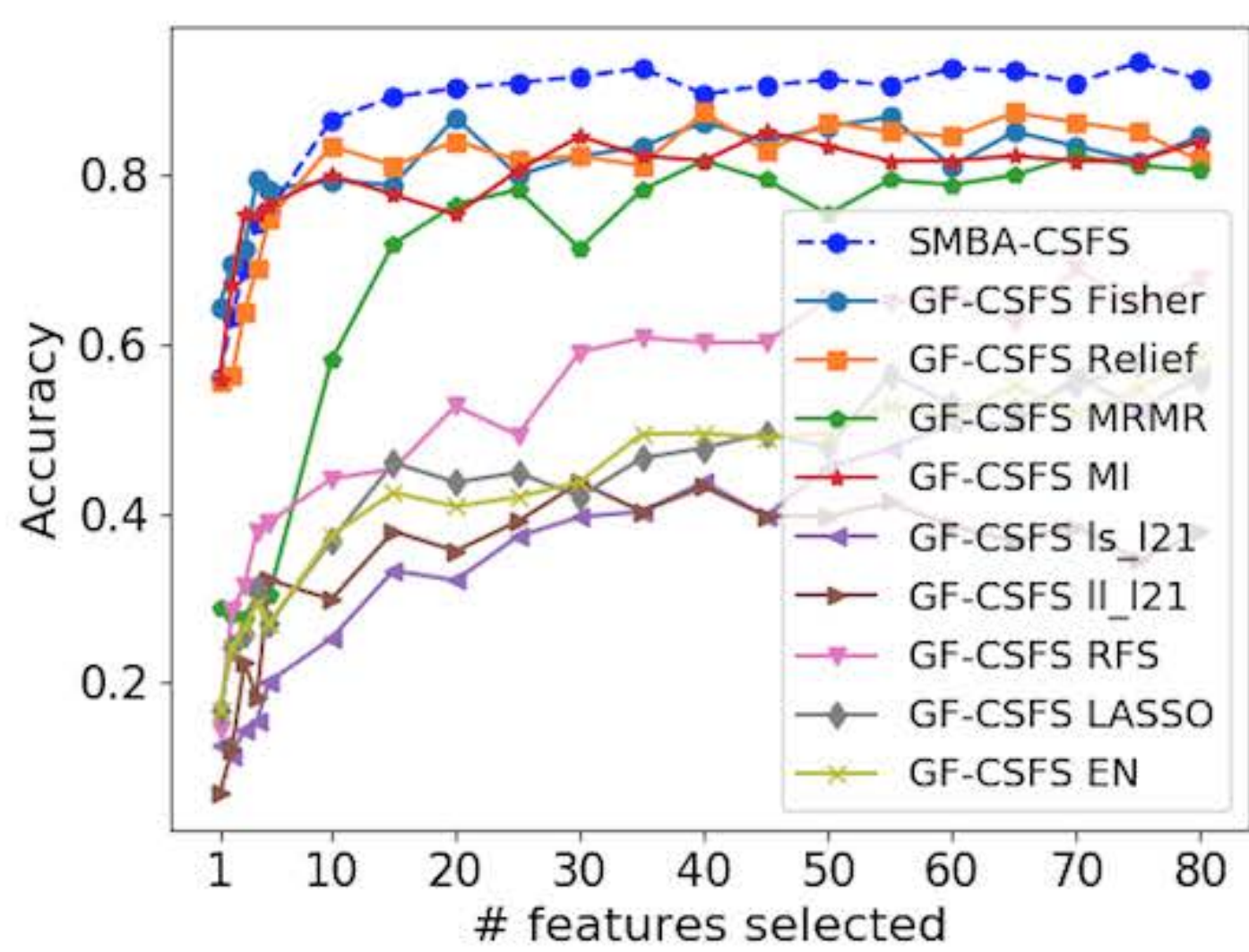
(h) CARCINOM (11)
