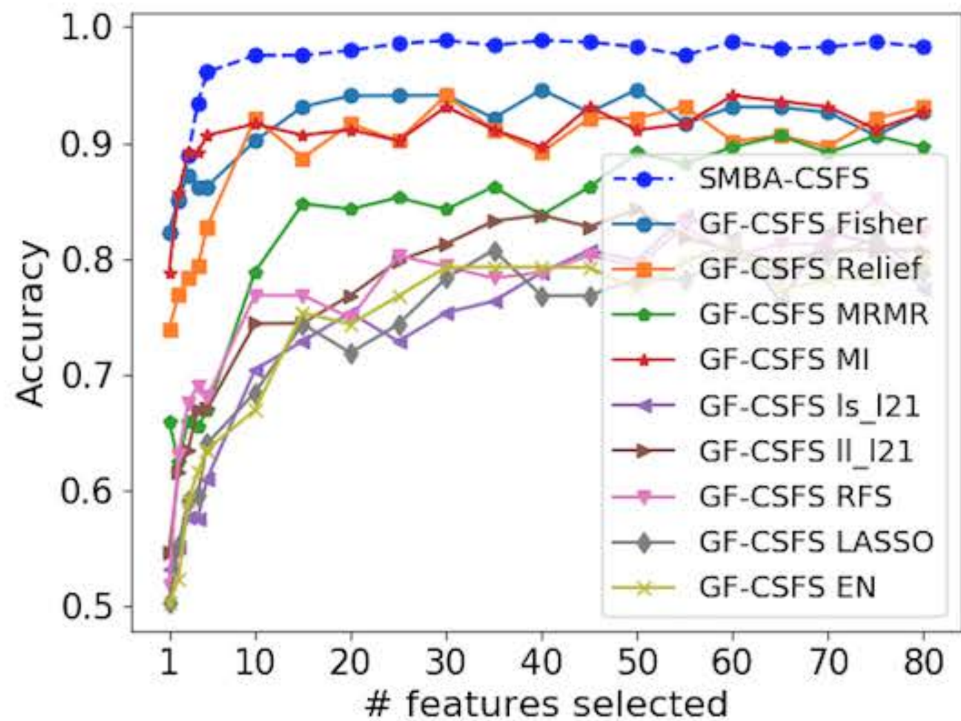
(e) LUNG_C (5)
