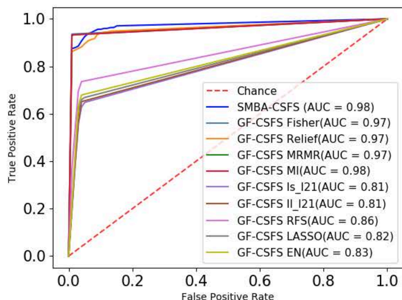
(h) CARCINOM (11)
