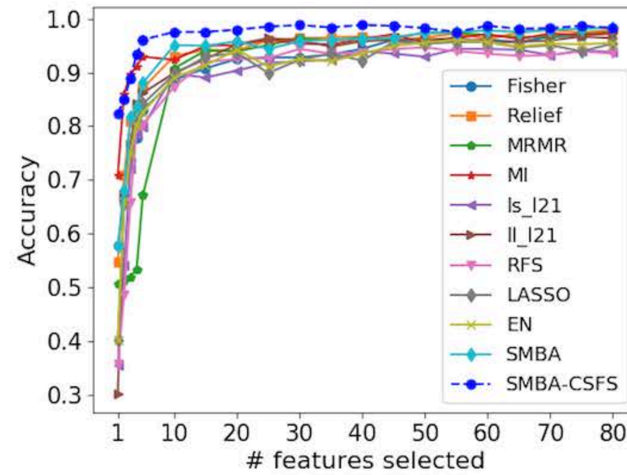
(e) LUNG_C (5)
