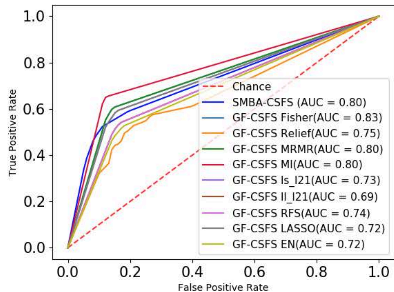
(d) GLIOMA (4)
