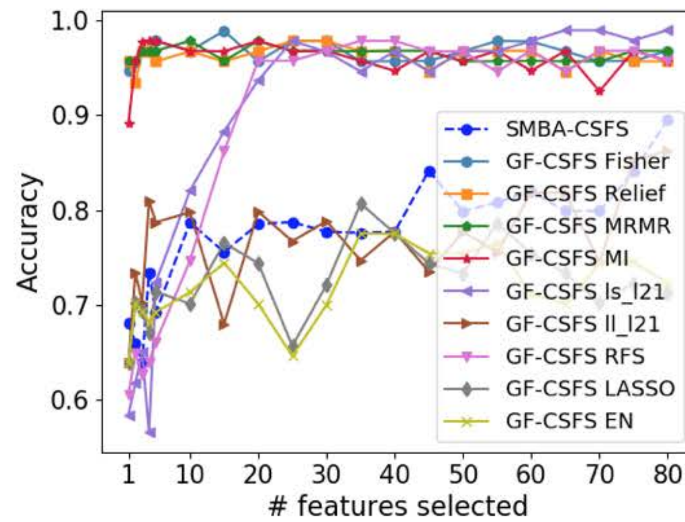
(b) LEUKEMIA (2)
