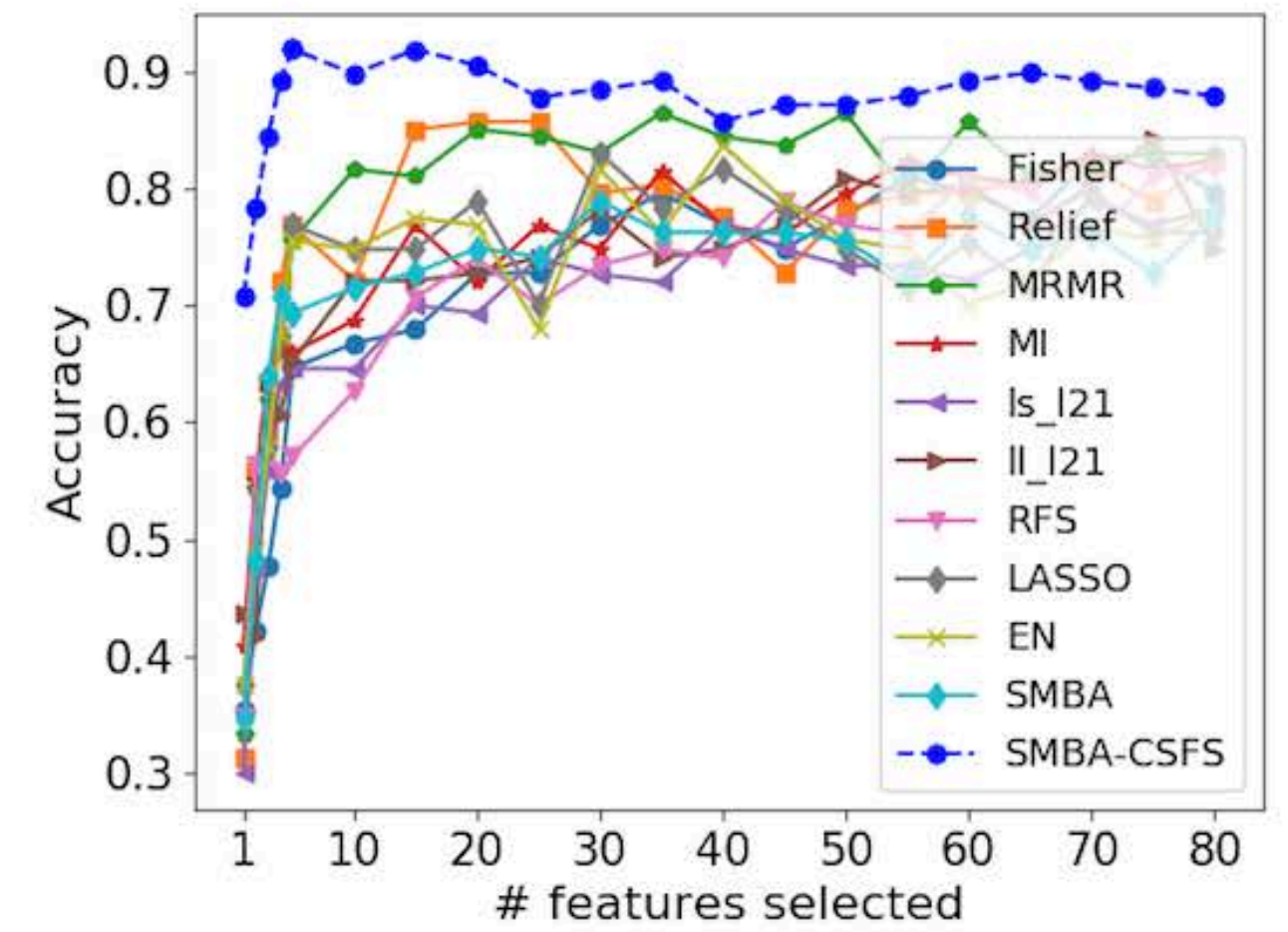
(f) LUNG_D (7)
