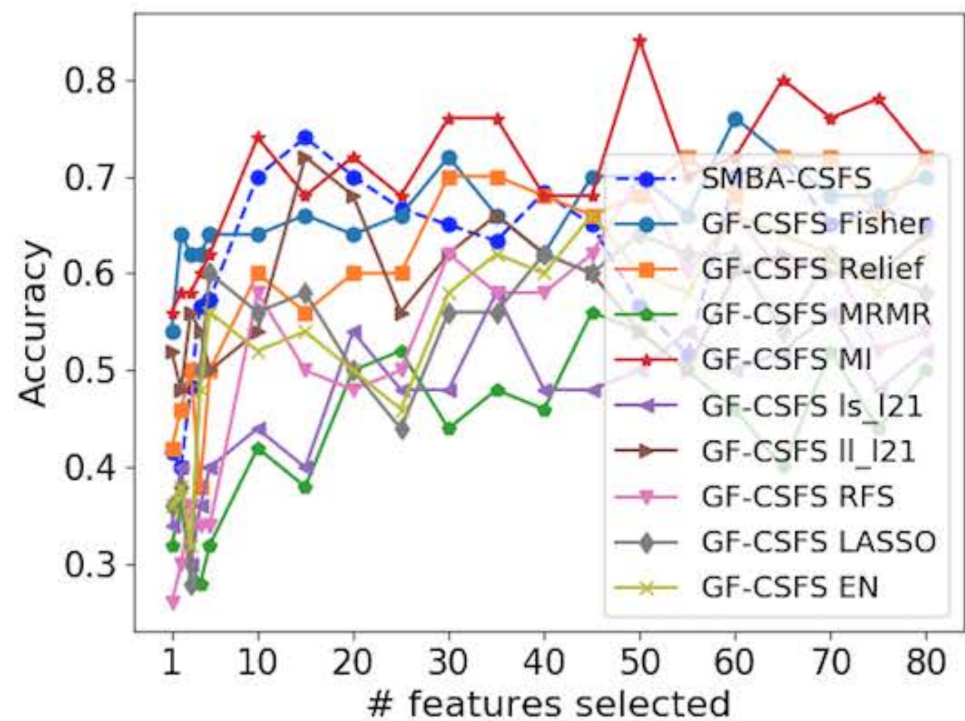
(d) GLIOMA (4)
