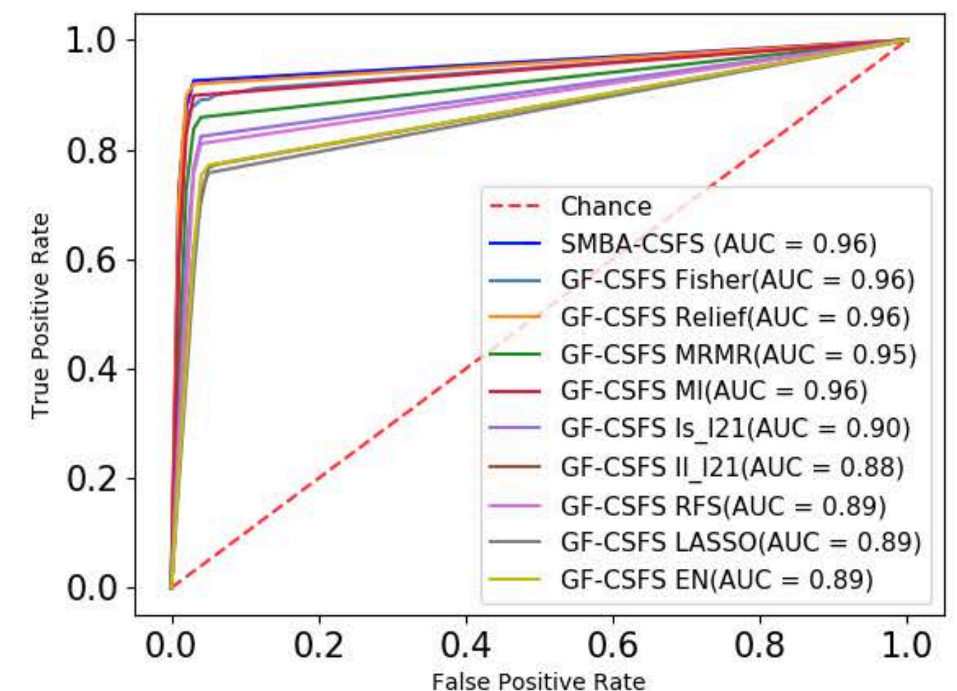
(f) LUNG_D (7)
