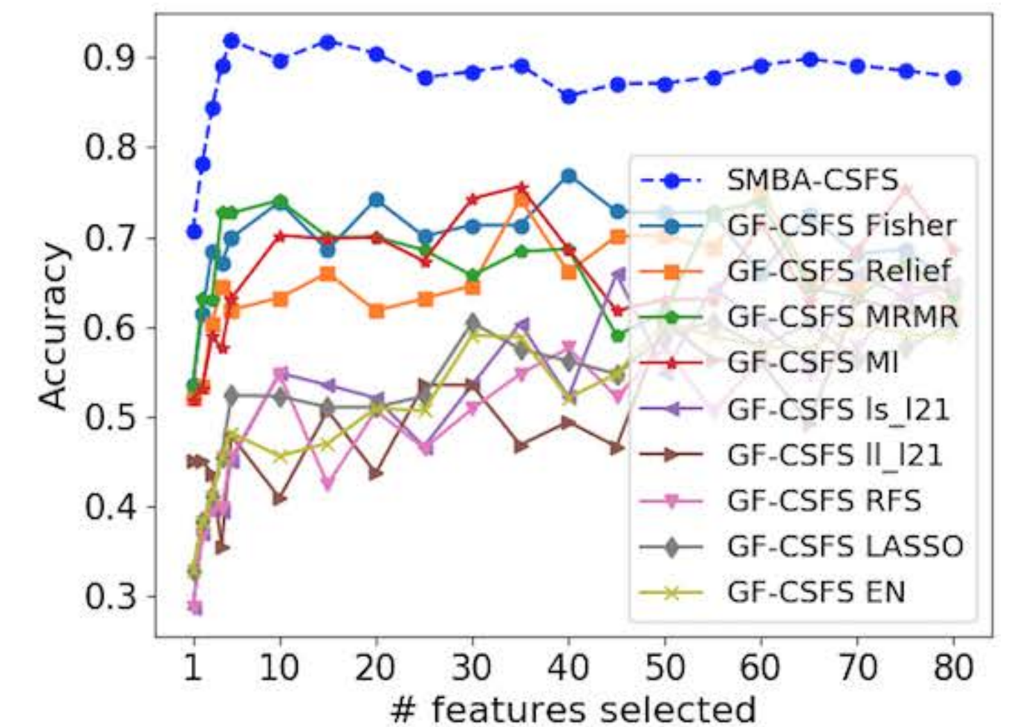
(f) LUNG_D (7)
