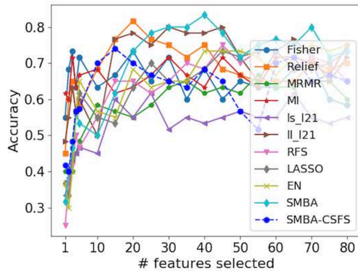
(d) GLIOMA (4)
