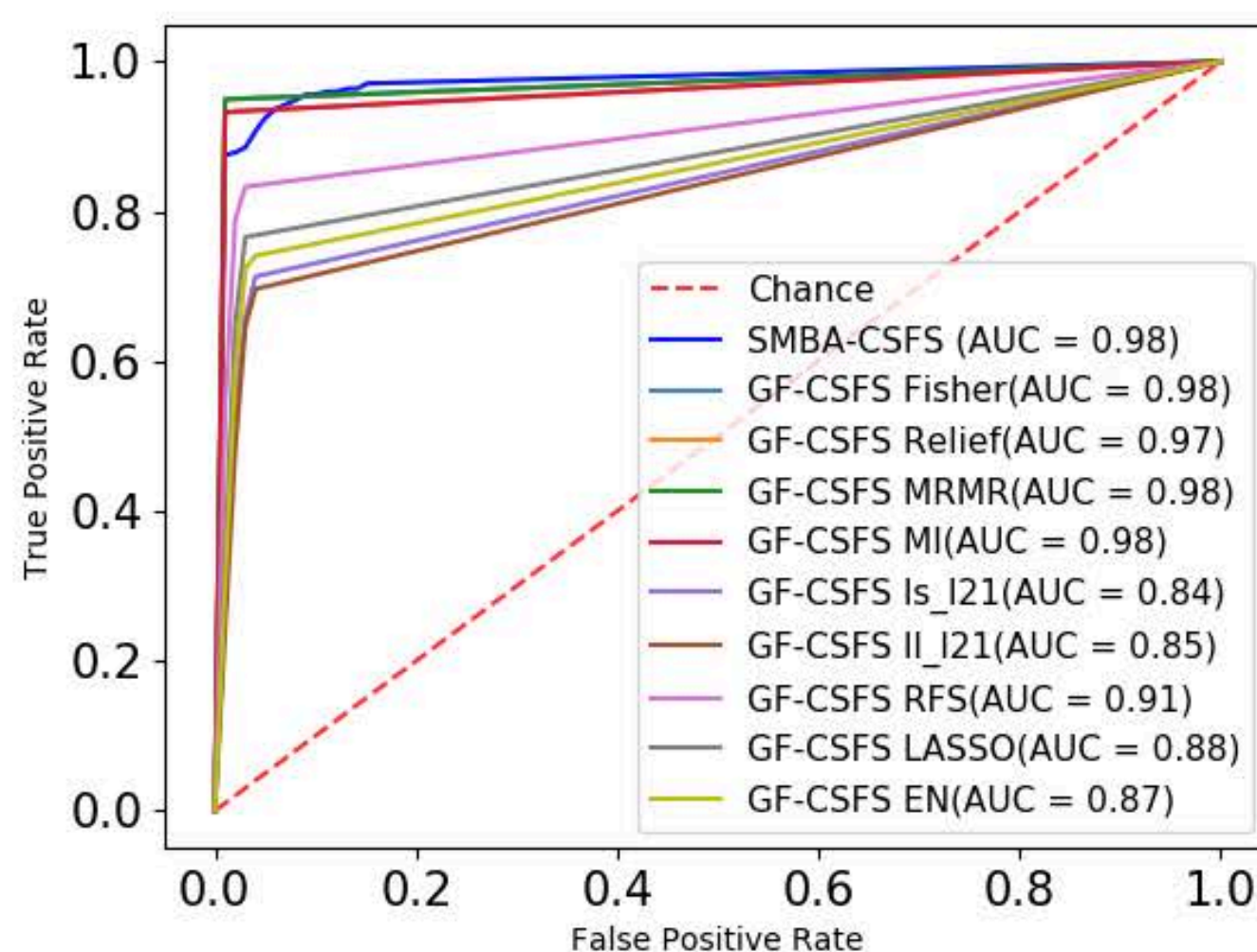
(h) CARCINOM (11)
