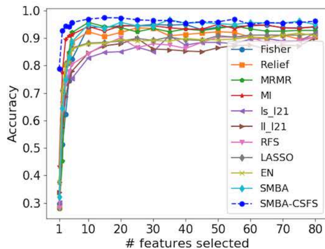
(g) DLBCL (9)
