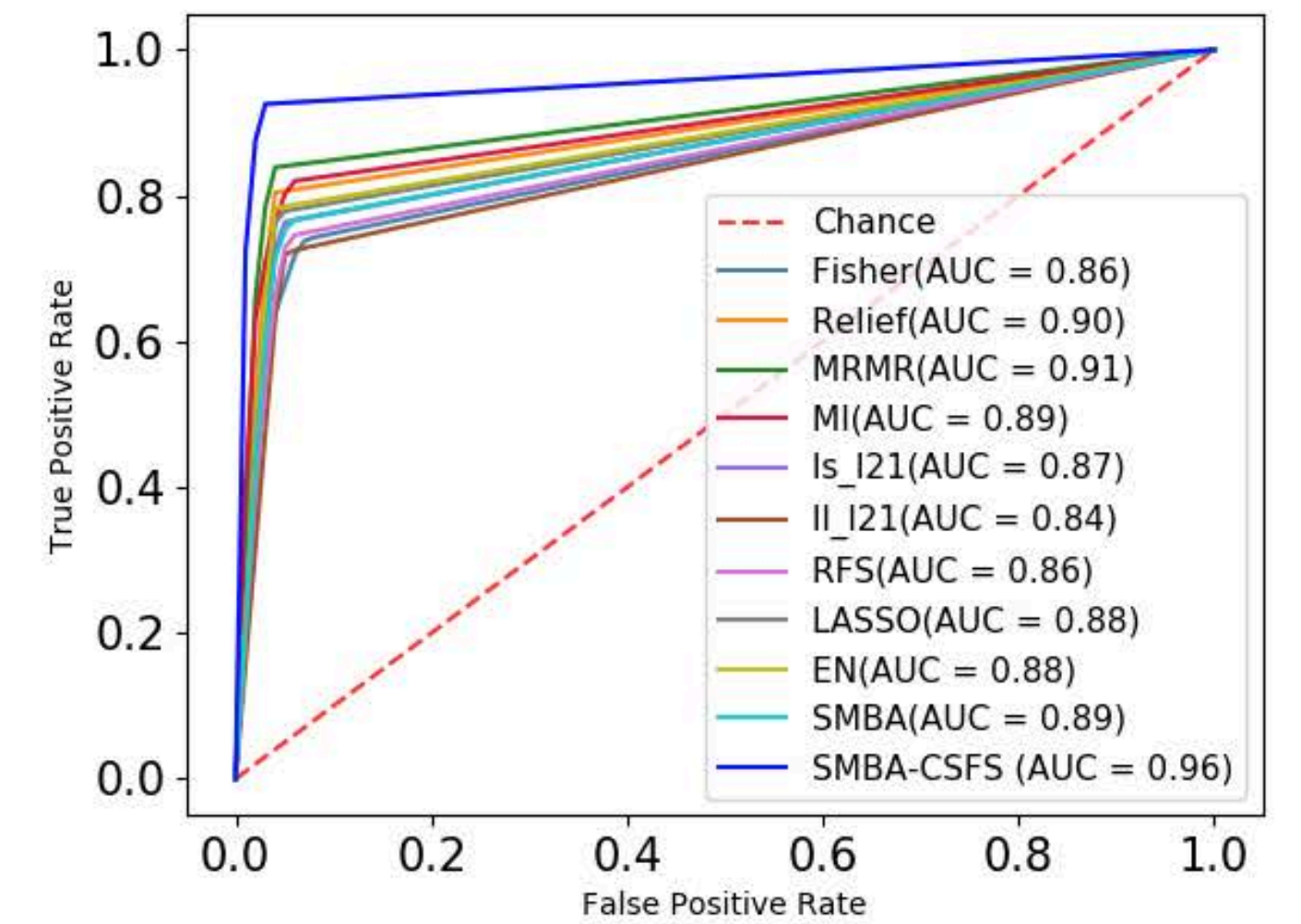
(f) LUNG_D (7)
