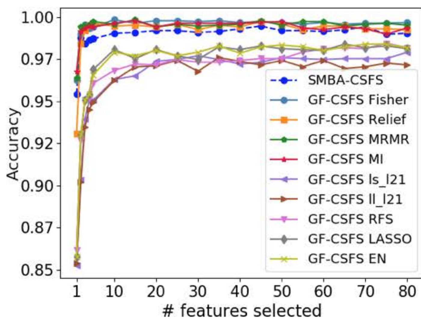
(g) DLBCL (9)
