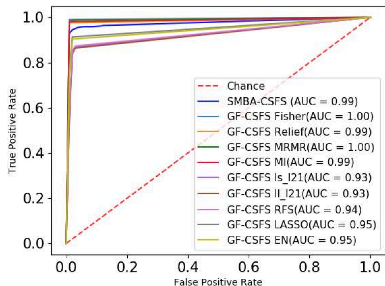
(g) DLBCL (9)
