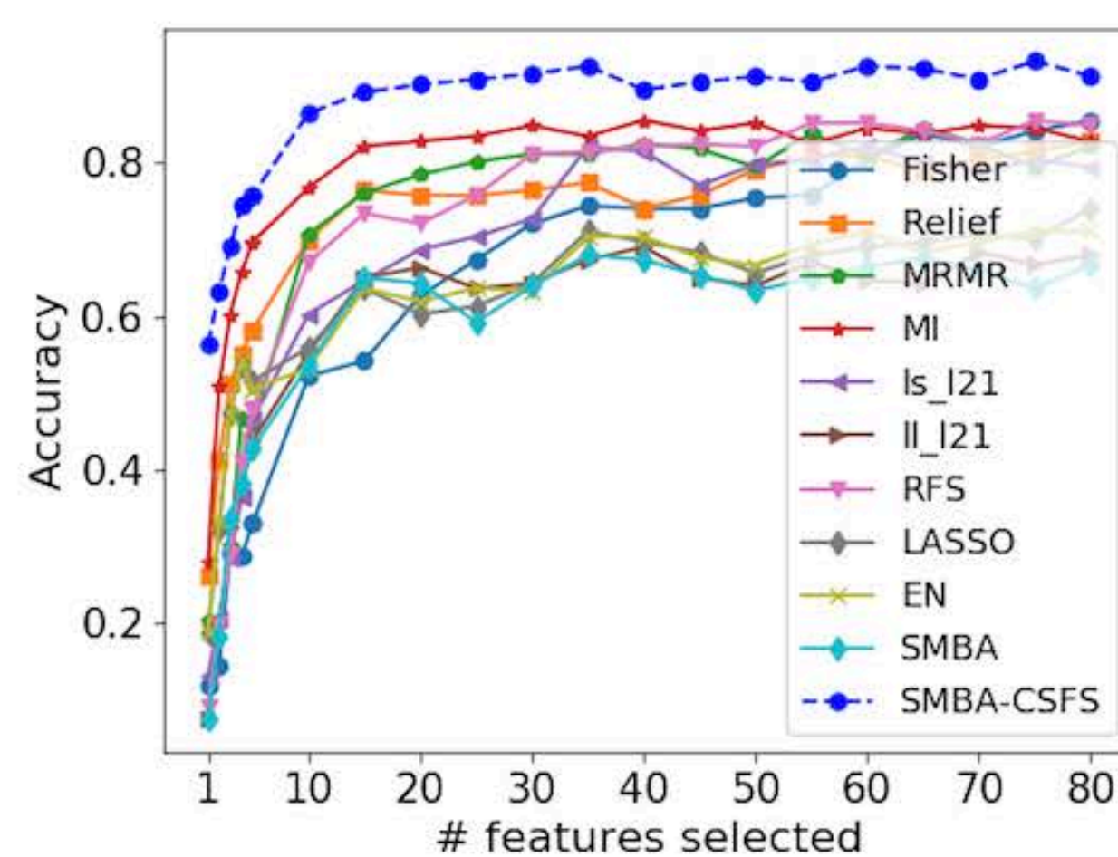
(h) CARCINOM (11)
