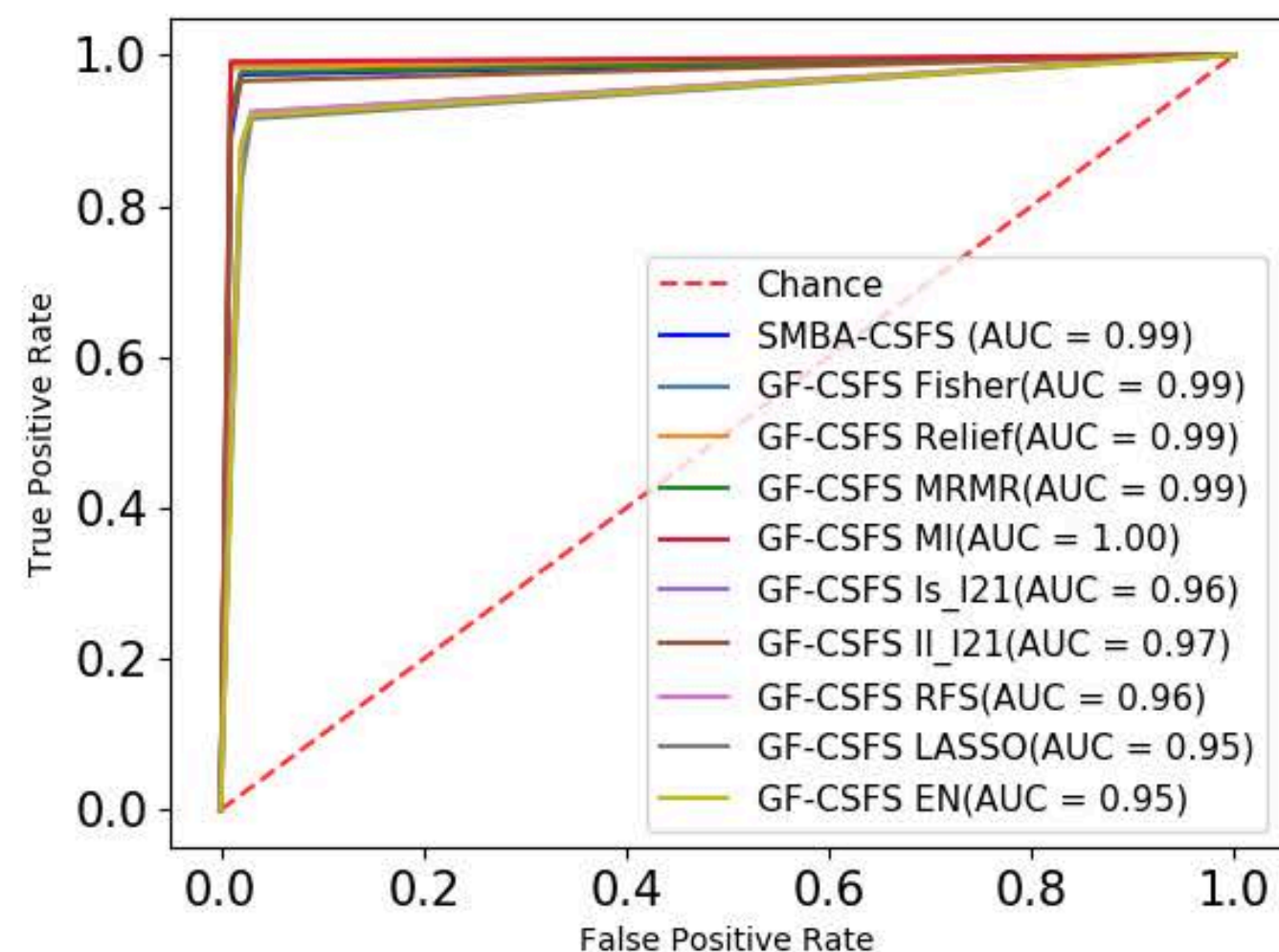
(e) LUNG_C (5)
