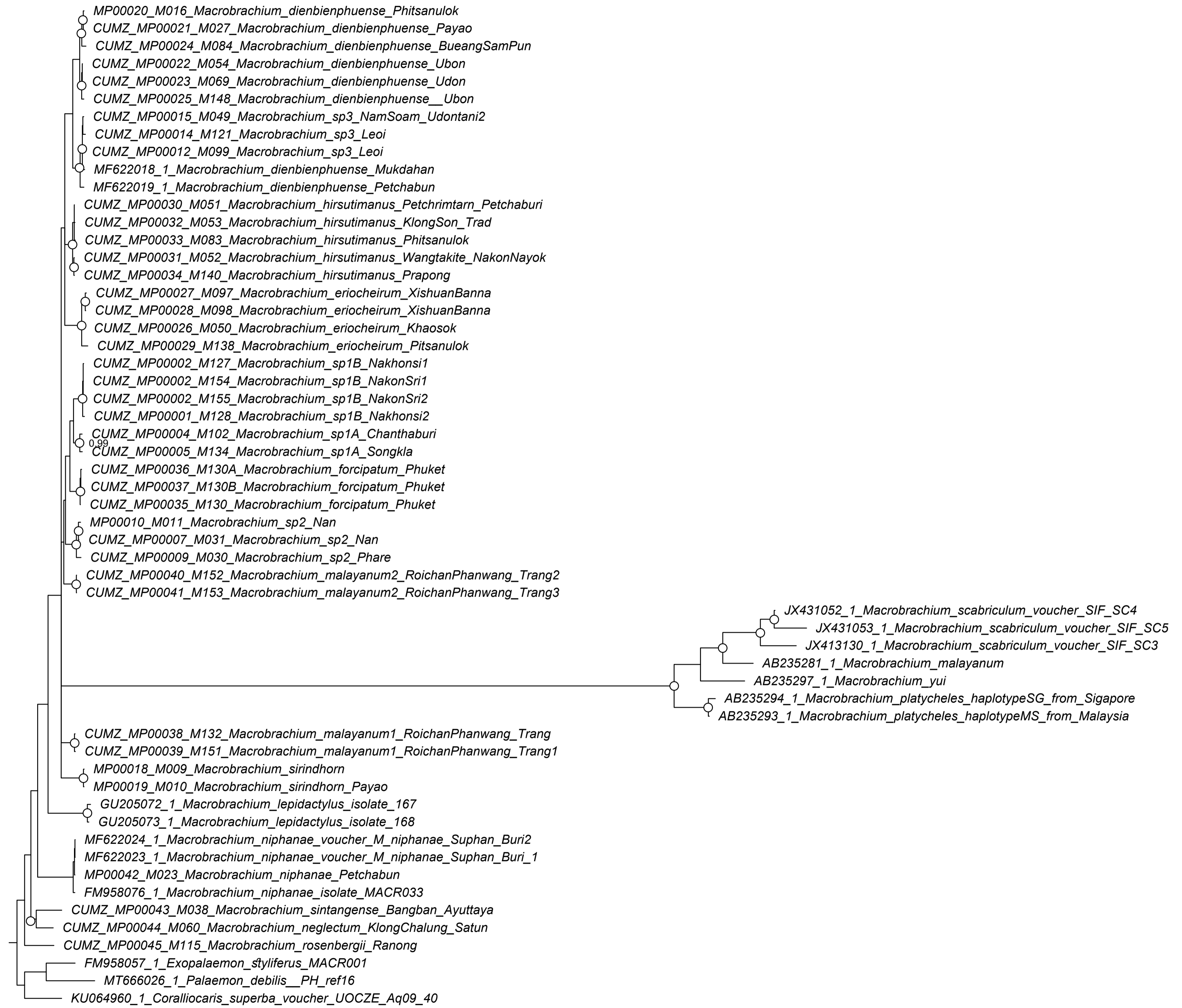
COI (N=57)
