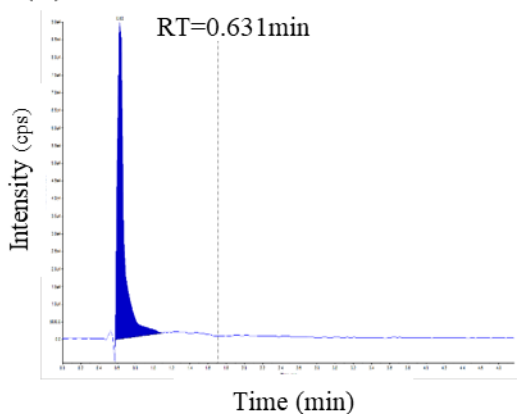
(E) 18:2 LPA
