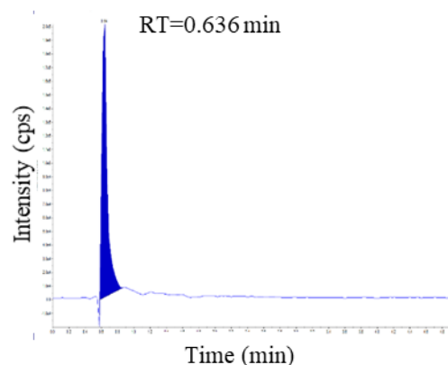
(D) 18:1 LPA
