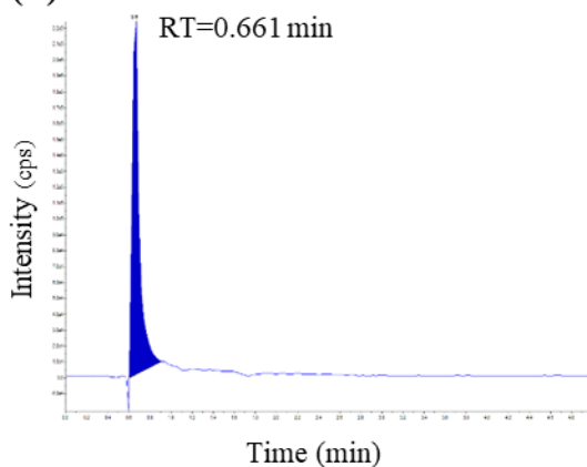
(E) 18:2 LPA
