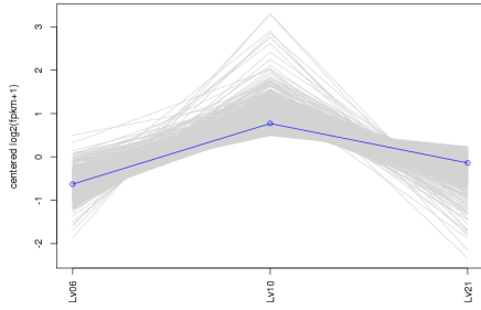
subcluster_4_log2_medianCentered_fpkm.matrix, 2391 trans
