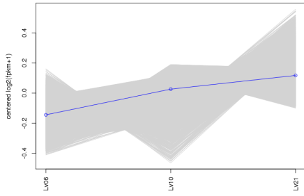
subcluster_4_log2_medianCentered_fpkm.matrix, 2391 trans
