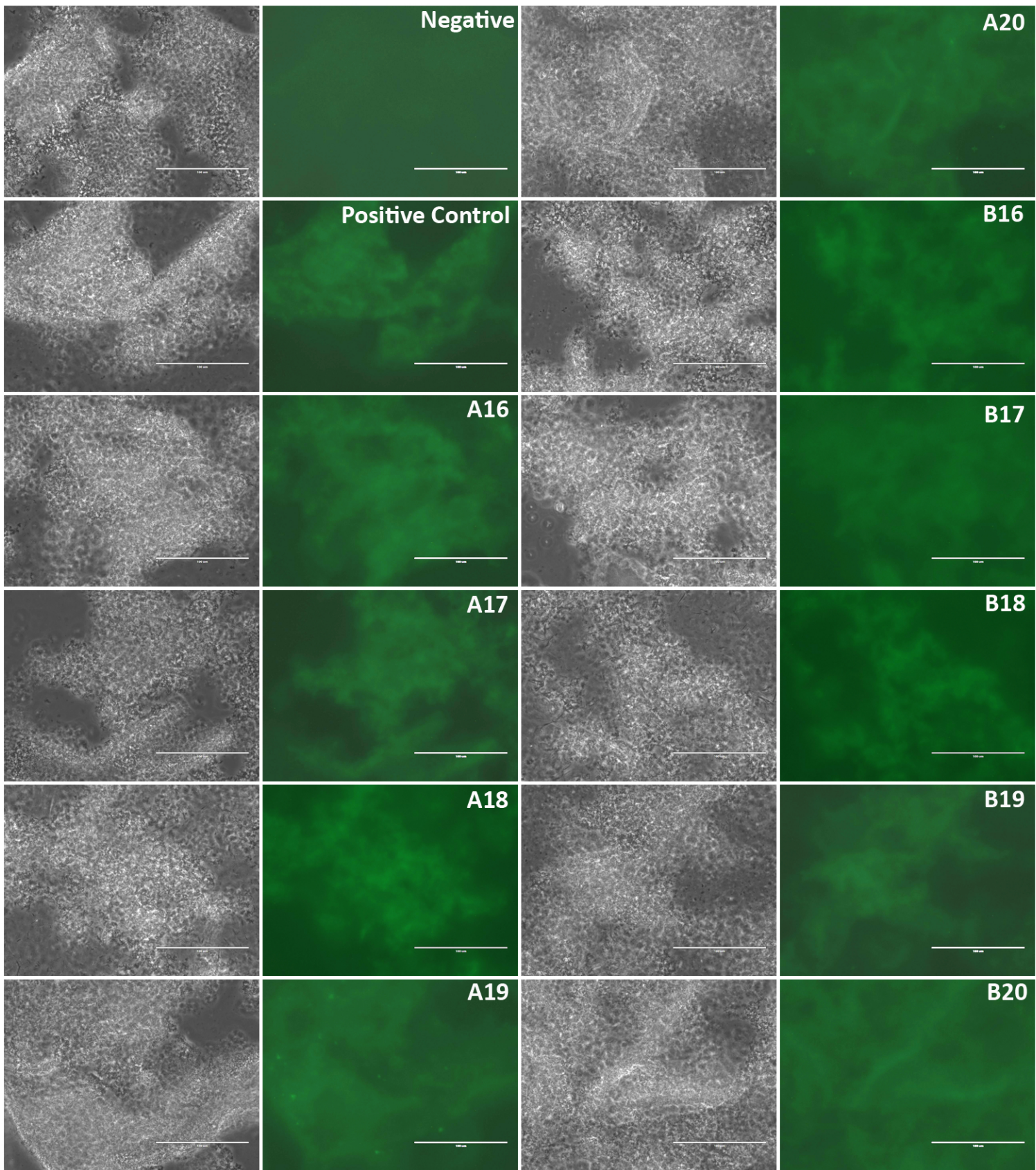
Fig. S8
