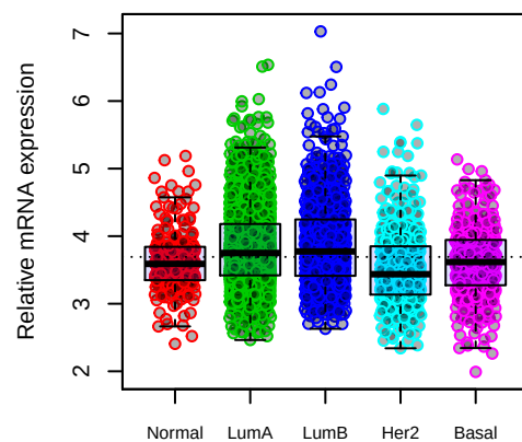
KIAA1429
