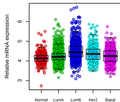
YTHDF1
