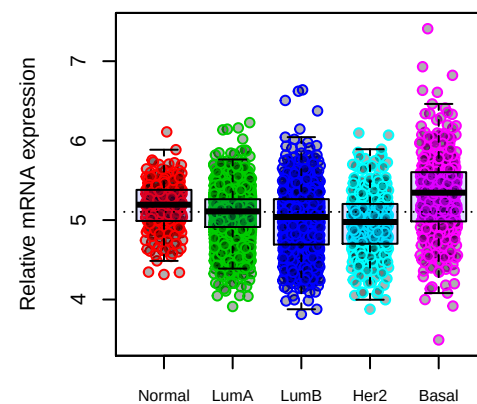
WTAP
