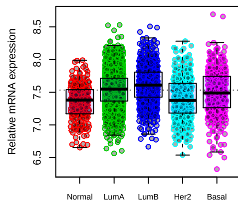
HNRNPC
