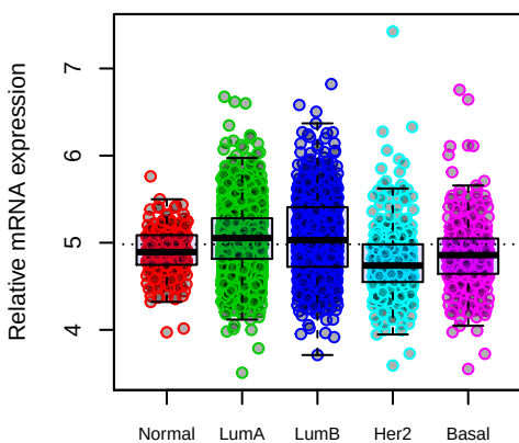
ALKBH5
