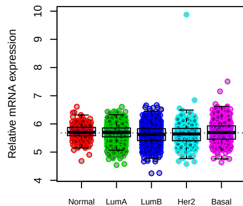
EIF3A
