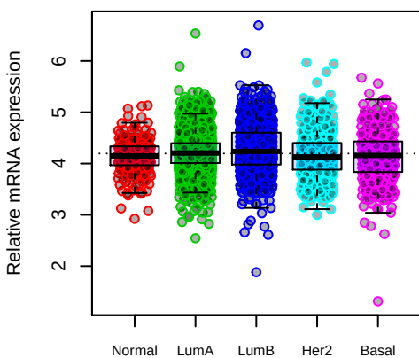
YTHDF3
