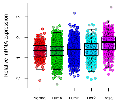
RBM15
