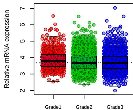
KIAA1429
