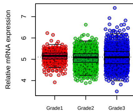
WTAP
