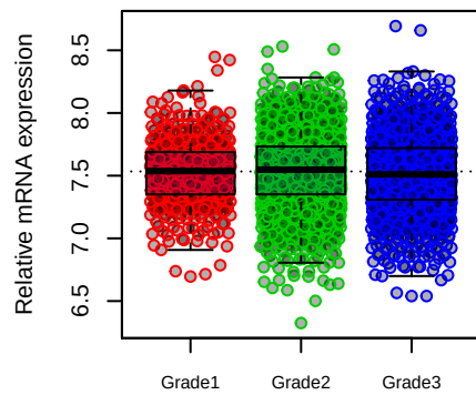
HNRNPC
