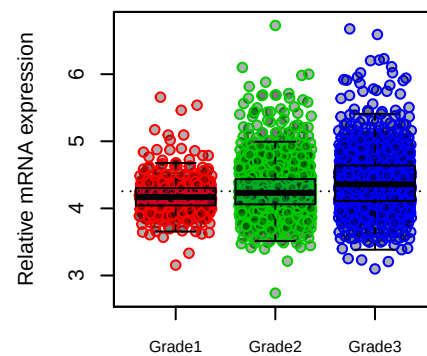
YTHDF1
