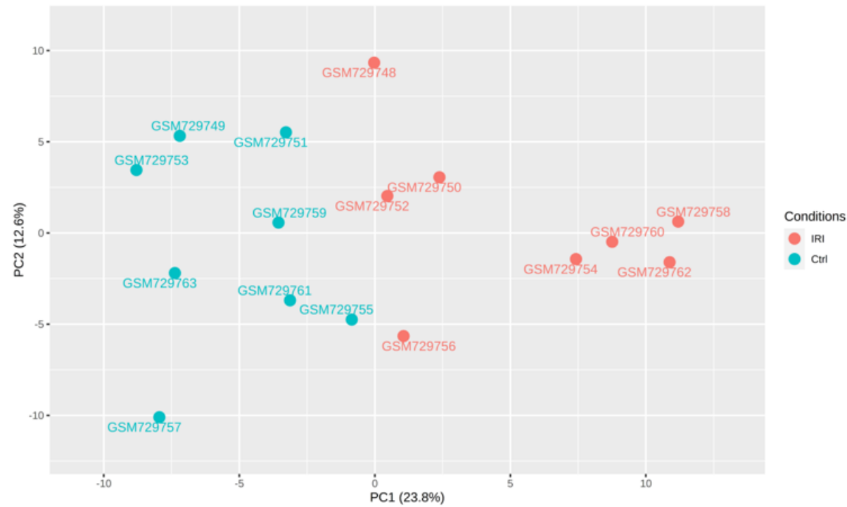
GSE29495
