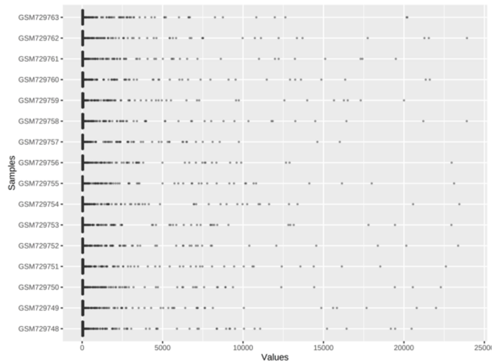
GSE39548
