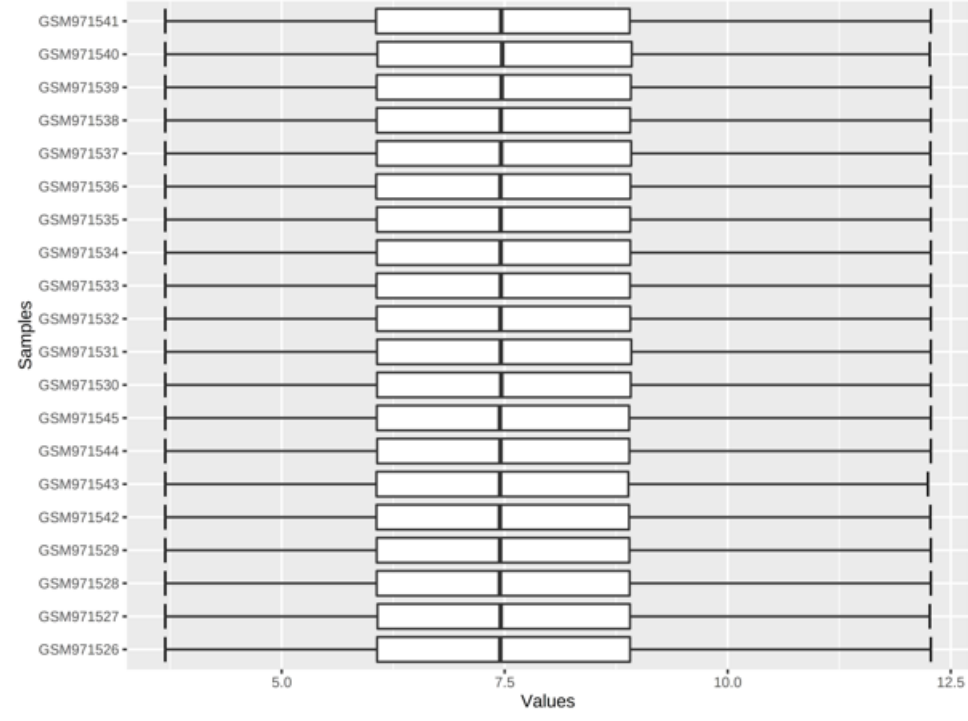
GSE39548
