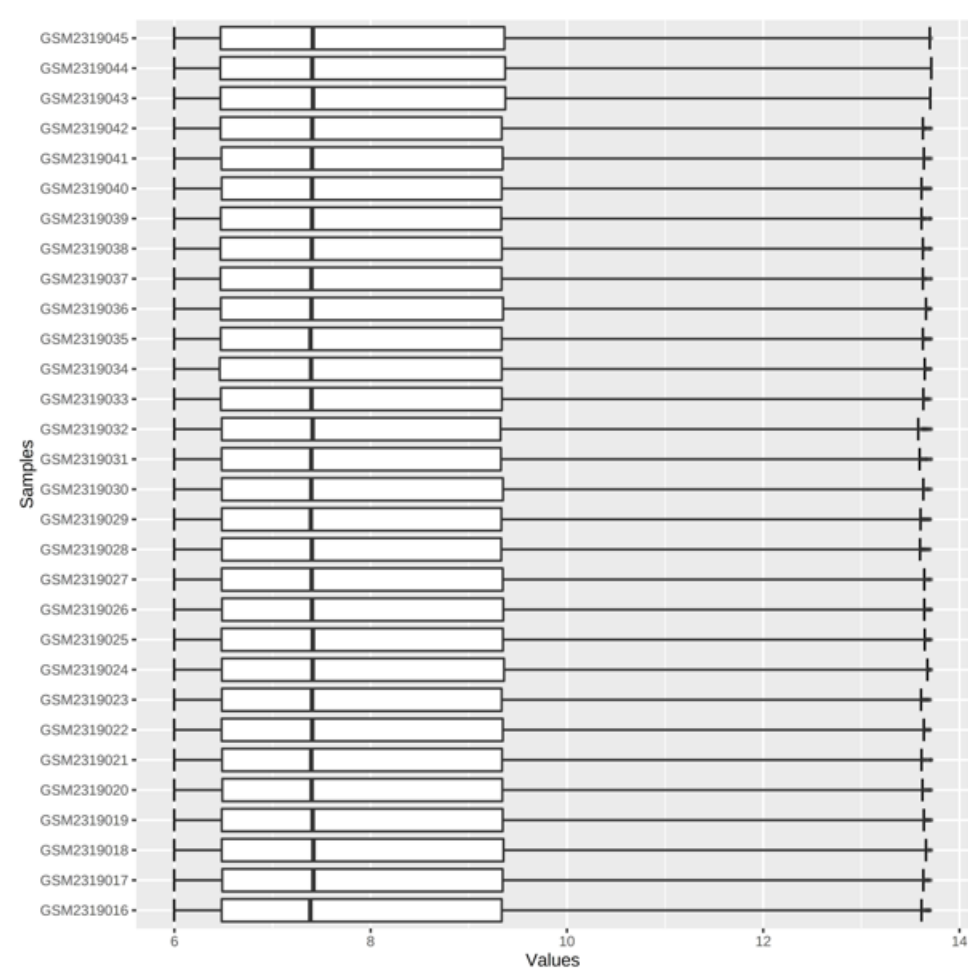
GSE87025
