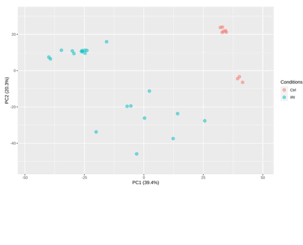
GSE87025
