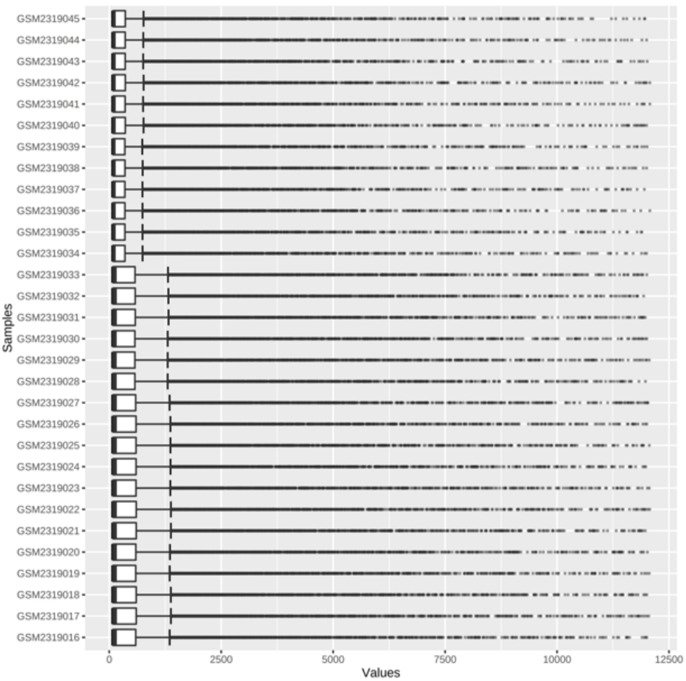
GSE87025
