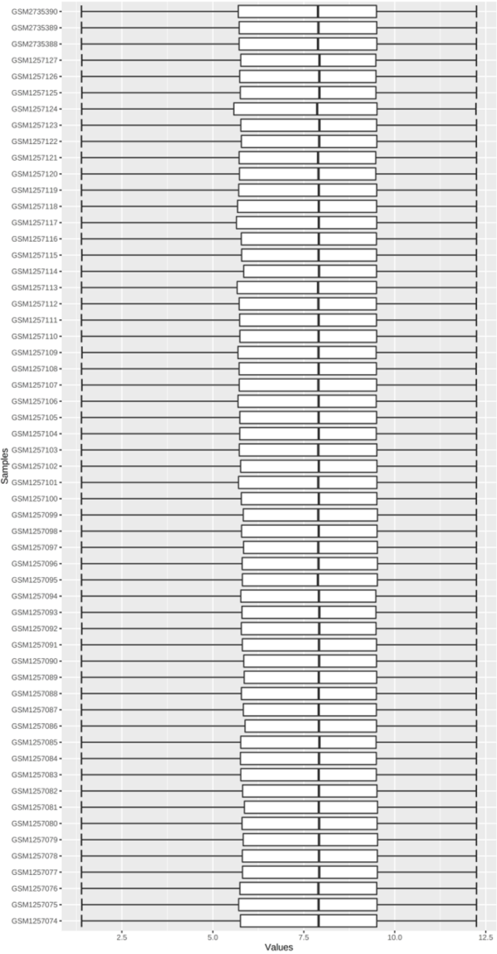
GSE52004
