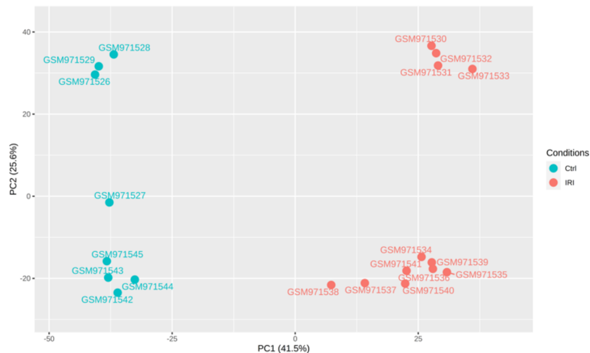
GSE39548
