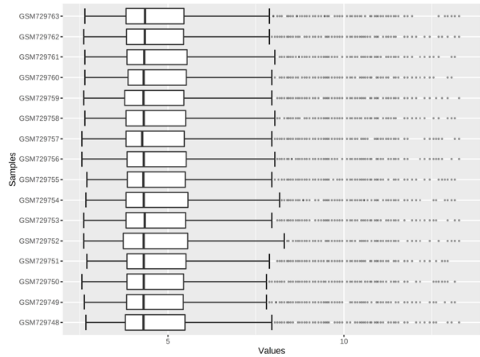
GSE29495
