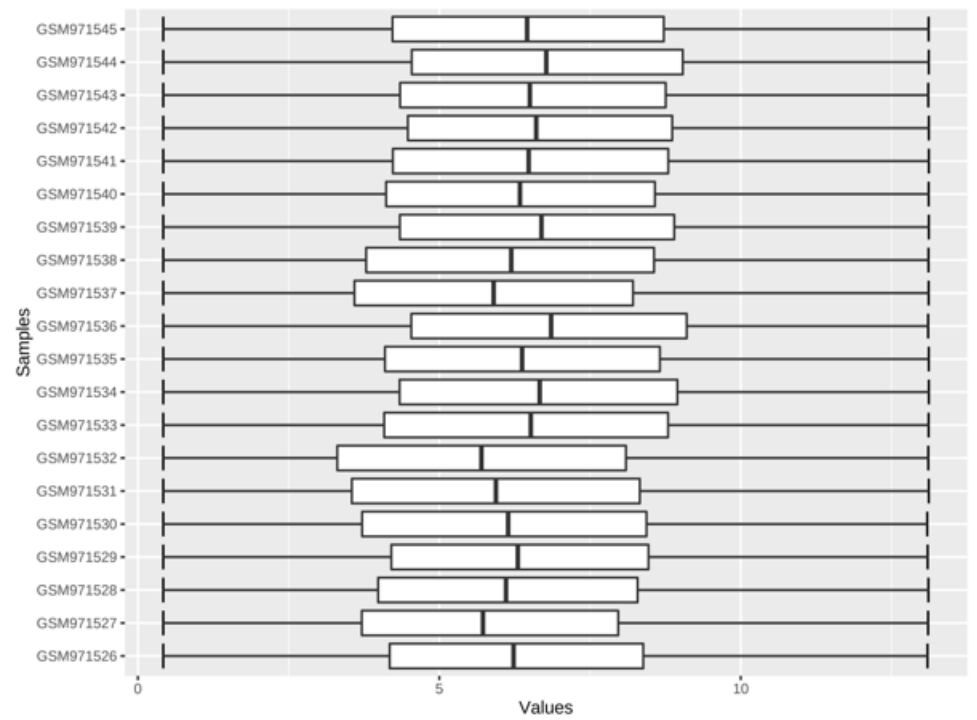
GSE87025
