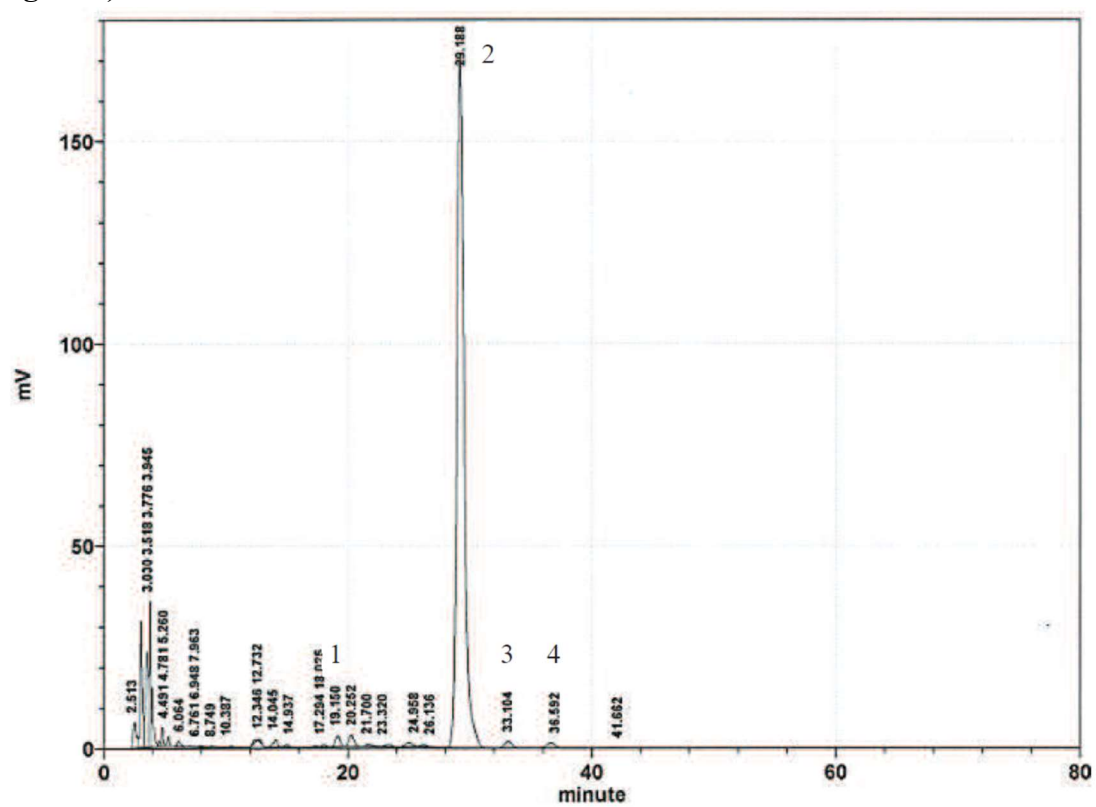
Fig. S2b) CF-2 HPLC
