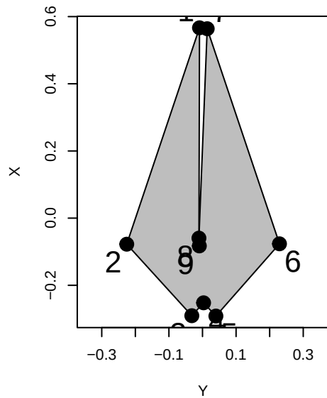
Tursiops_truncatus
