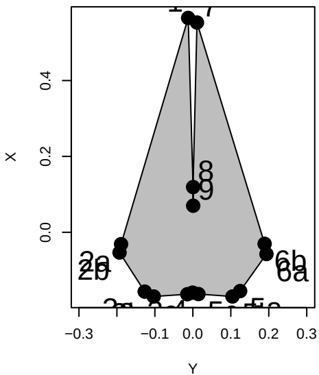
Balaenoptera acutorostrata
