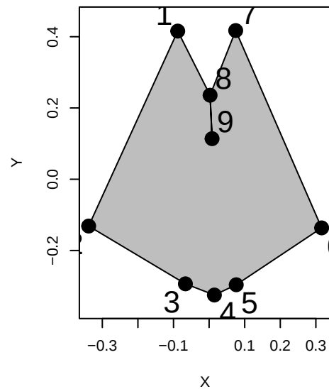
Tursiops_aduncus
