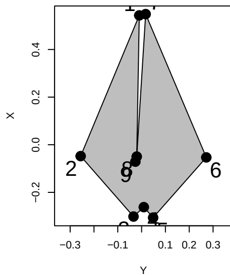
Feresa_attenuata
