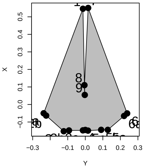
Eubalaena glacialis
