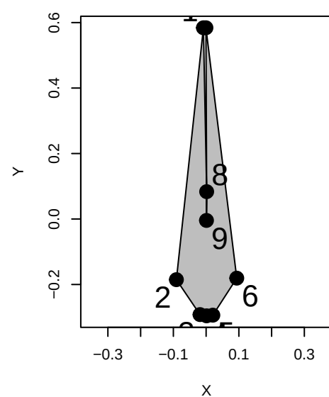
Balaenoptera_borealis
