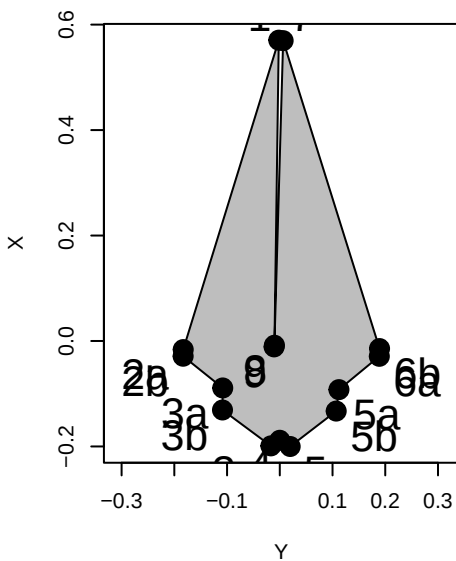
Stenella_coeruleoalba
