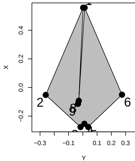
Grampus_griseus
