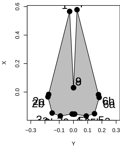
Balaenoptera_physalus
