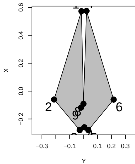
Tursiops_aduncus
