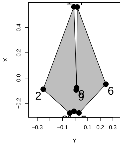
Orcinus_orca
