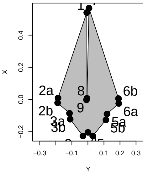
Sousa_teuszii
