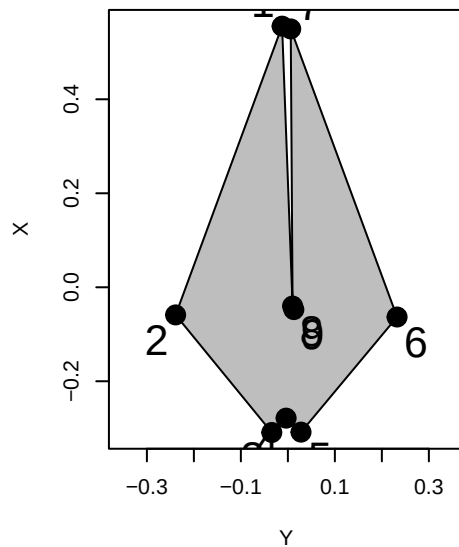
Lagenorhynchus_australis
