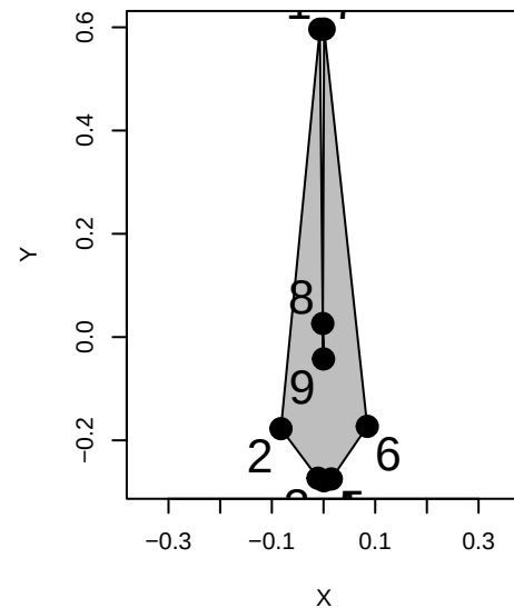
Megaptera_novaeangliae
