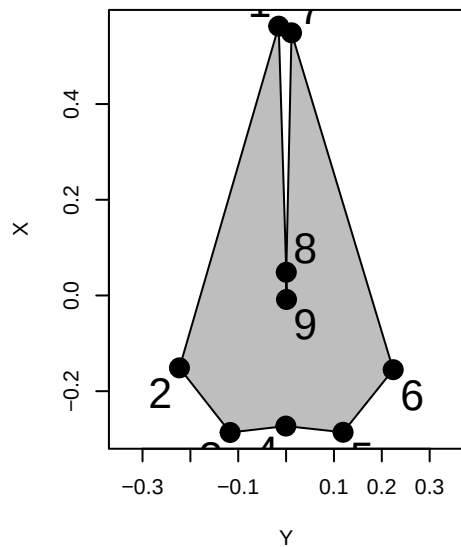
Balaenoptera acutorostrata
