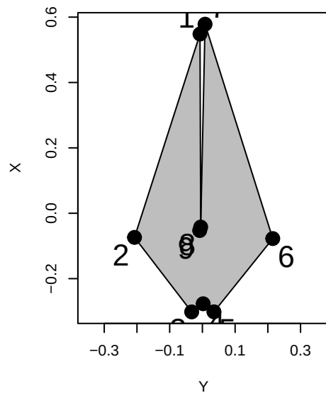
Sousa_teuszii
