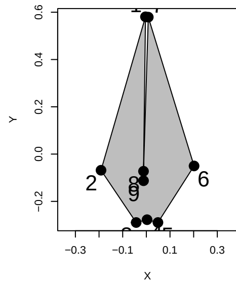
Neophocaena_asiaeorientalis
