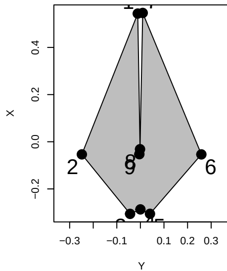
Phocoenoides dalli
