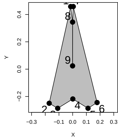
Balaenoptera acutorostrata
