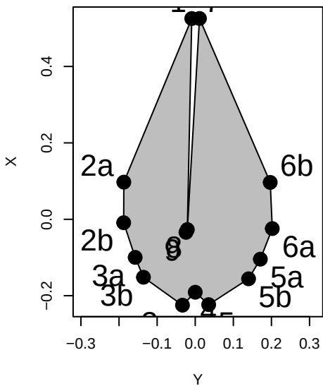
Delphinapterus_leucas
