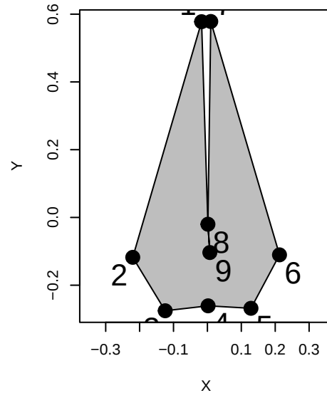
Steno_bredanensis
