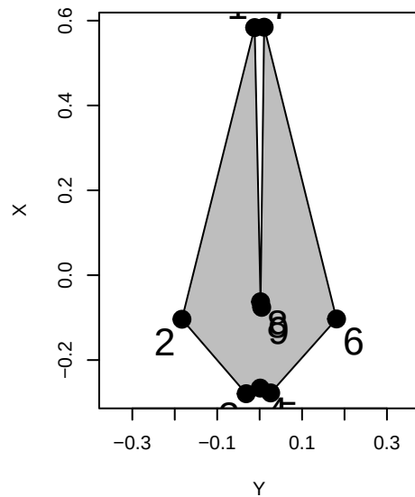
Sousa_plumbea
