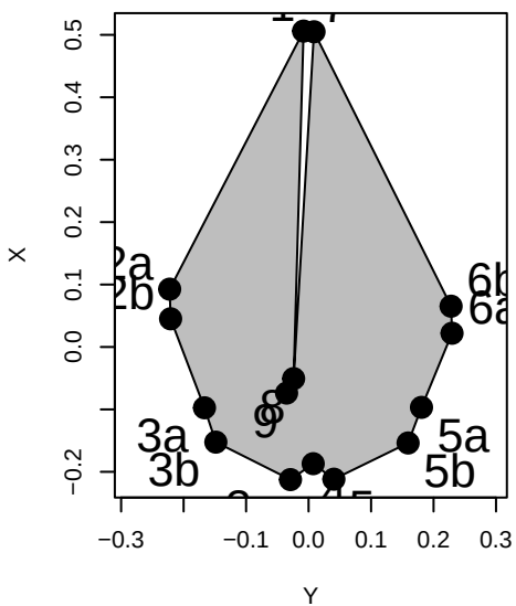
Monodon_monoceros
