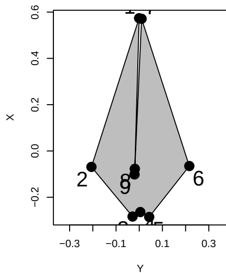
Lagenorhynchus_obscurus
