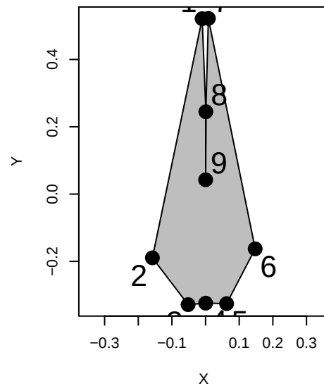
Lagenorhynchus_acutus
