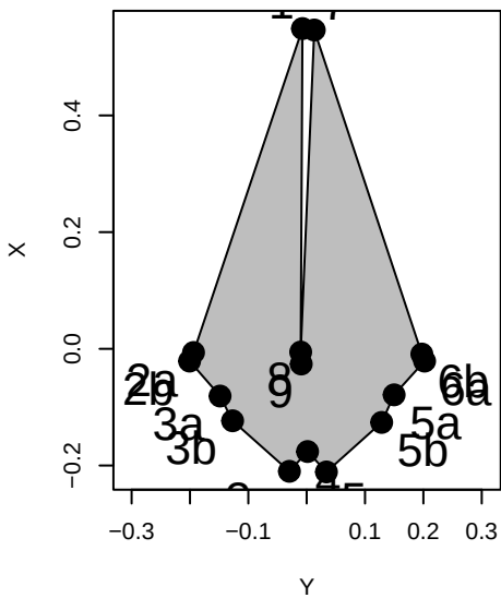
Tursiops_truncatus
