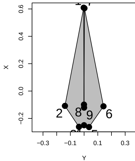
Pontoporia blainvillei
