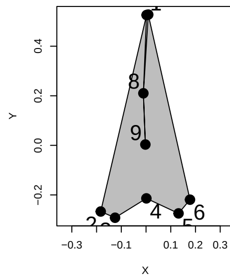
Stenella_attenuata
