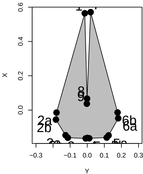
Balaenoptera_edeni
