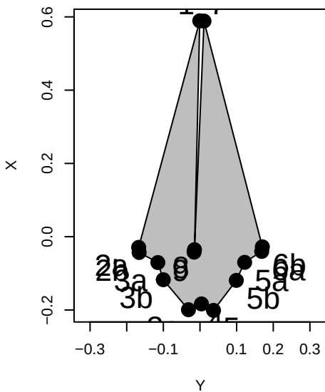
Stenella_attenuata
