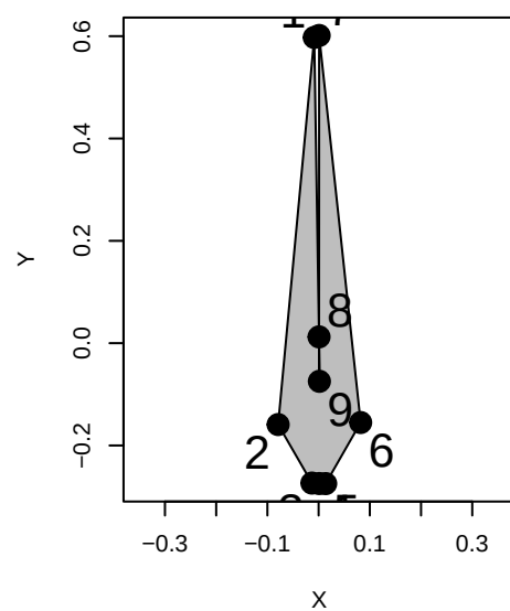
Eschrichtius_robustus
