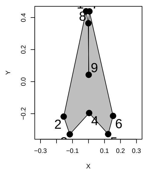
Balaenoptera_physalus
