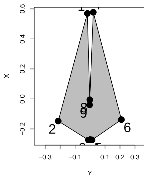
Balaenoptera_edeni
