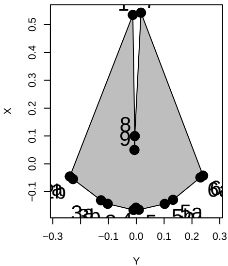
Eubalaena australis
