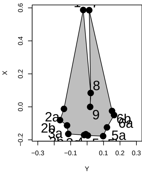
Eschrichtius_robustus
