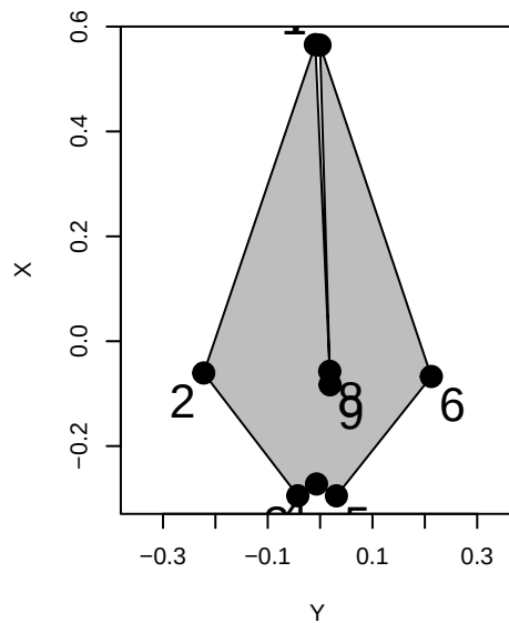
Lagenorhynchus_obliquidens
