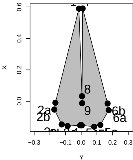
Balaenoptera_musculus
