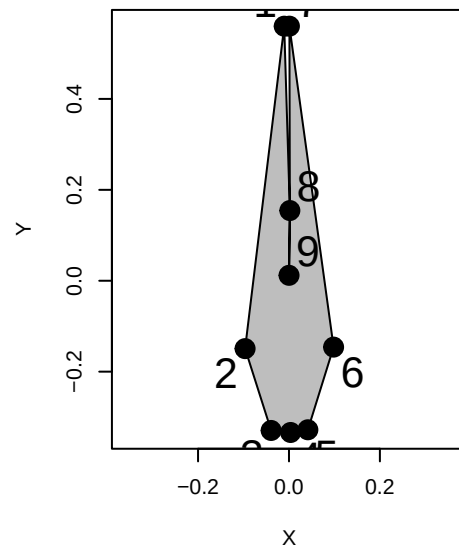
Globicephala_macrorhynchus
