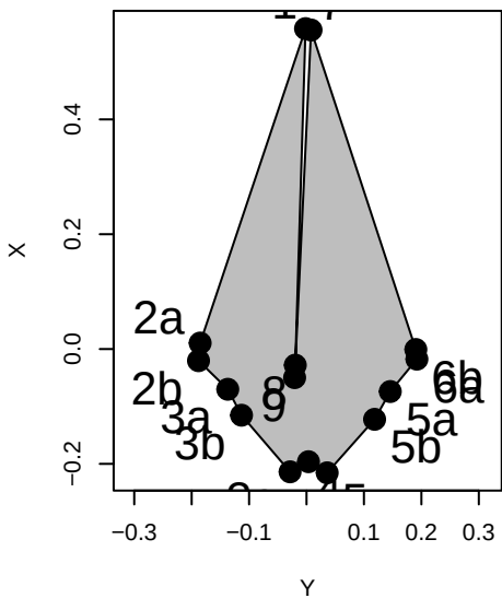
Lagenorhynchus_obscurus
