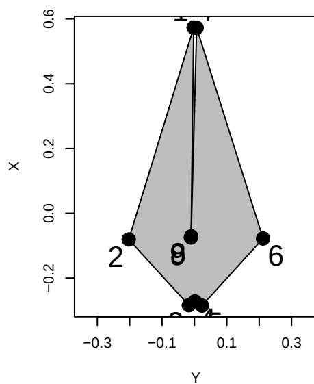
Stenella_coeruleoalba
