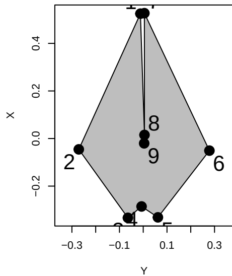
Neophocaena_asiaeorientalis
