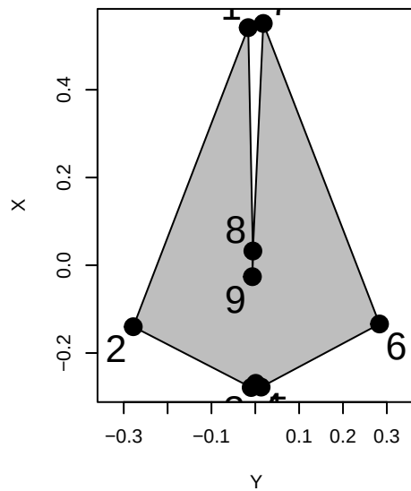
Eubalaena australis
