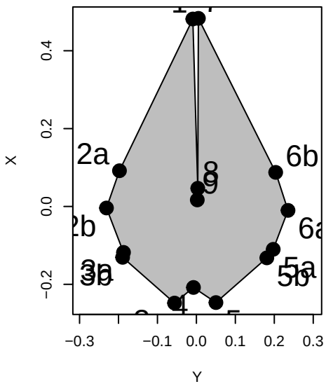
Neophocaena_asiaeorientalis
