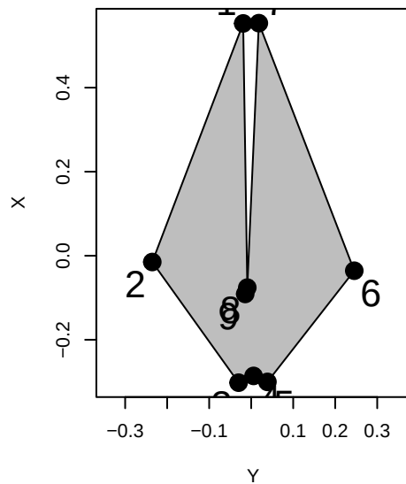
Lagenorhynchus_cruciger
