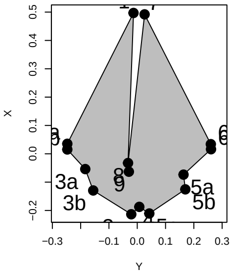
Globicephala_macrorhynchus
