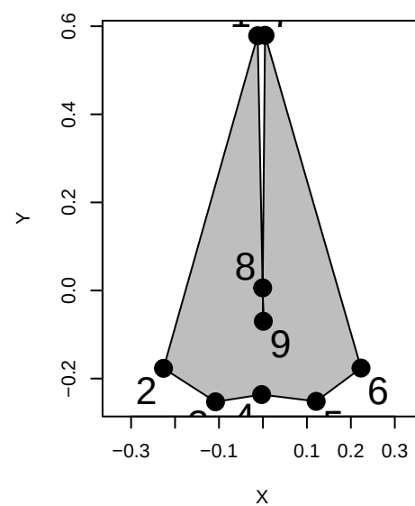
Mesoplodon perrini
