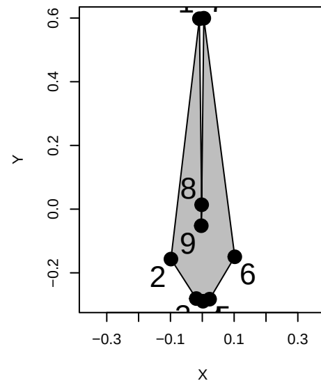
Lagenorhynchus_albirostris
