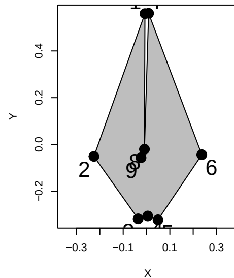
Phocoena_sinus
