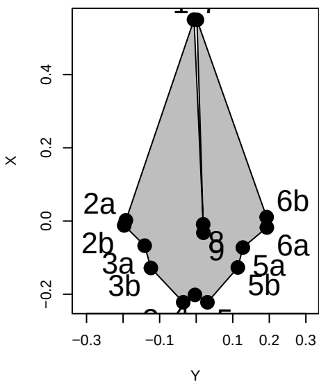
Lagenorhynchus_obliquidens
