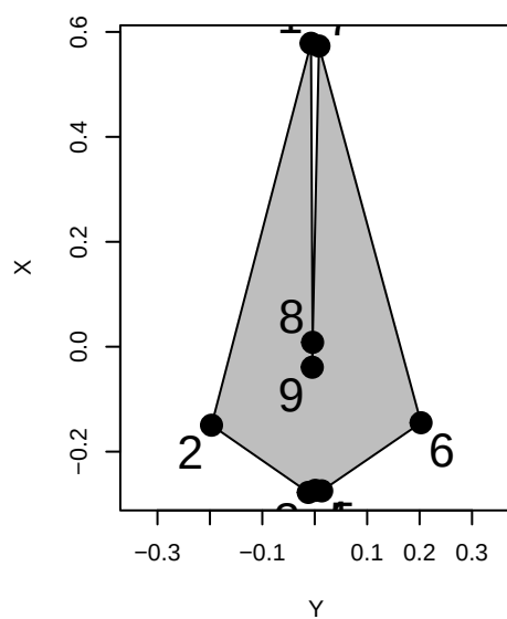
Balaenoptera_borealis
