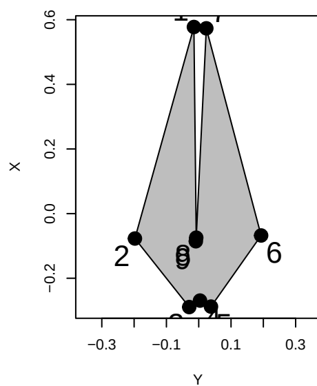
Sousa_sahuensis
