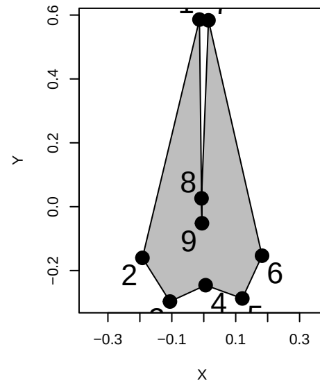
Monodon_monoceros
