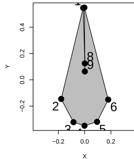
Pseudorca_crassidens
