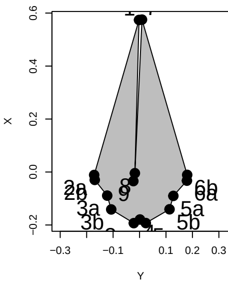
Mesoplodon perrini
