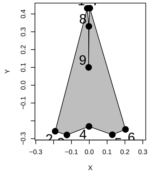
Eubalaena australis
