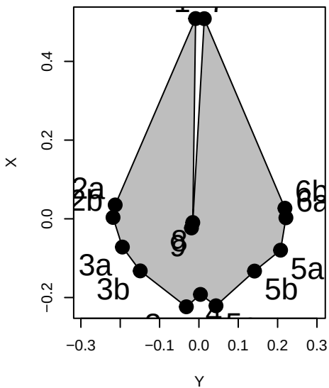
Pseudorca_crassidens
