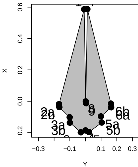
Sousa_plumbea
