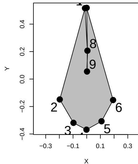
Orcinus_orca
