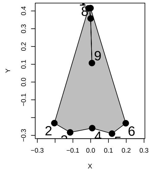
Eubalaena glacialis
