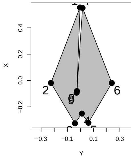
Globicephala_melas
