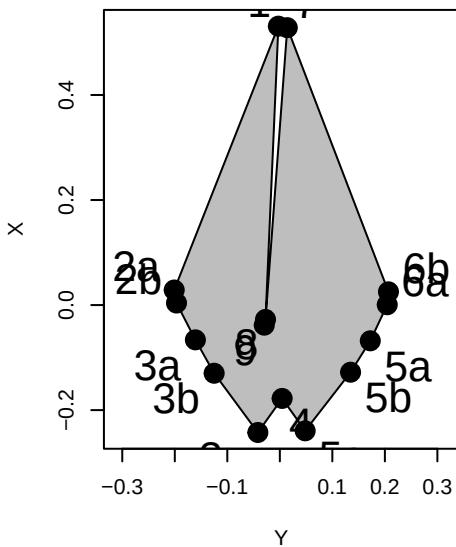
Globicephala_melas
