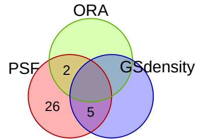
vesalius_exp_5
