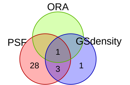
vesalius_exp_4
