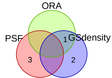
vesalius_exp_6
