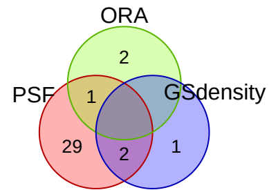
vesalius_exp_2
