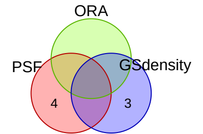
vesalius_exp_4
