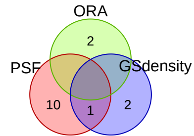
vesalius_exp_3
