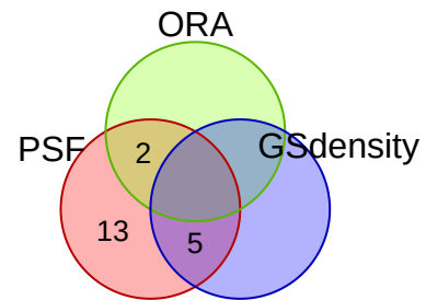
vesalius_exp_9
