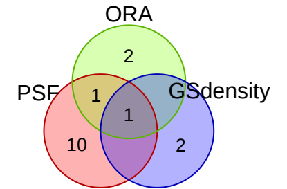
vesalius_exp_8
