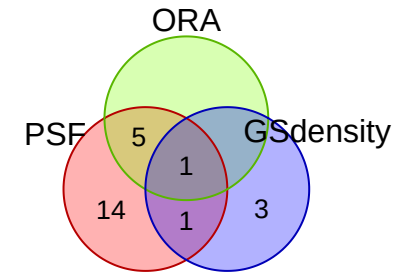
vesalius_exp_8
