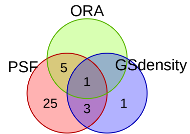
vesalius_exp_1
