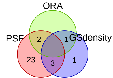
vesalius_exp_7
