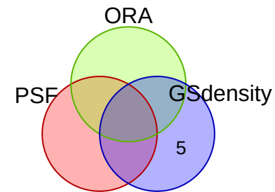
vesalius_exp_11
