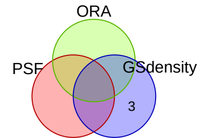
vesalius_exp_12
