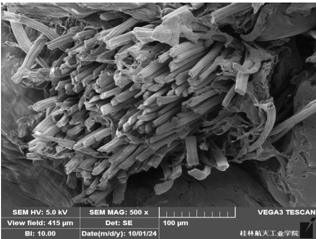
SEM image 155°C-160°C
